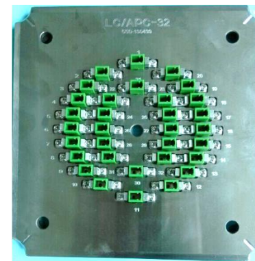
32 port
