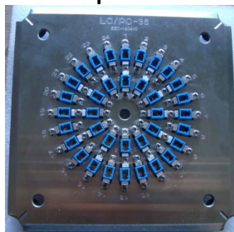
36 port
