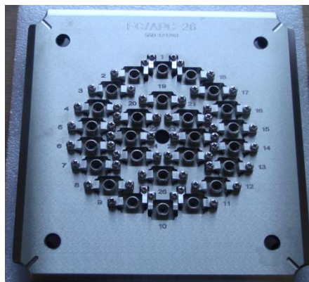
26 port
