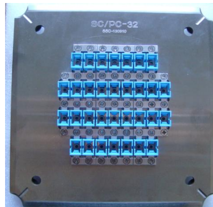
32 port
