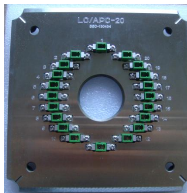
20 port
