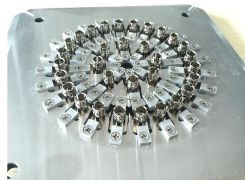
32 port
