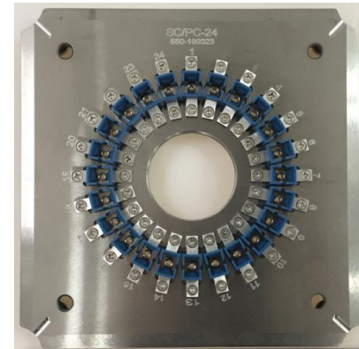
24 port
